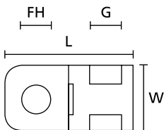
CTAM-serie (bovenaanzicht)
